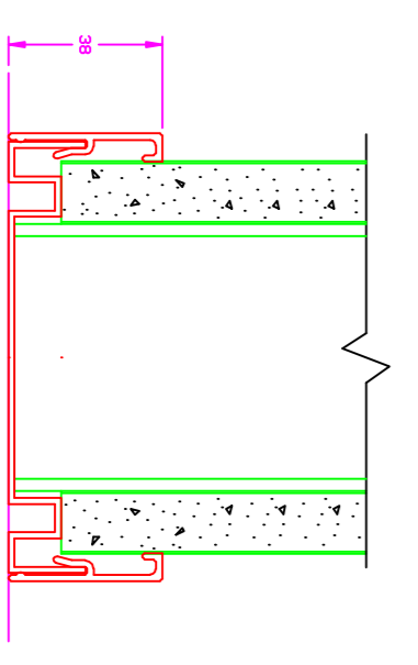
Section D-D
